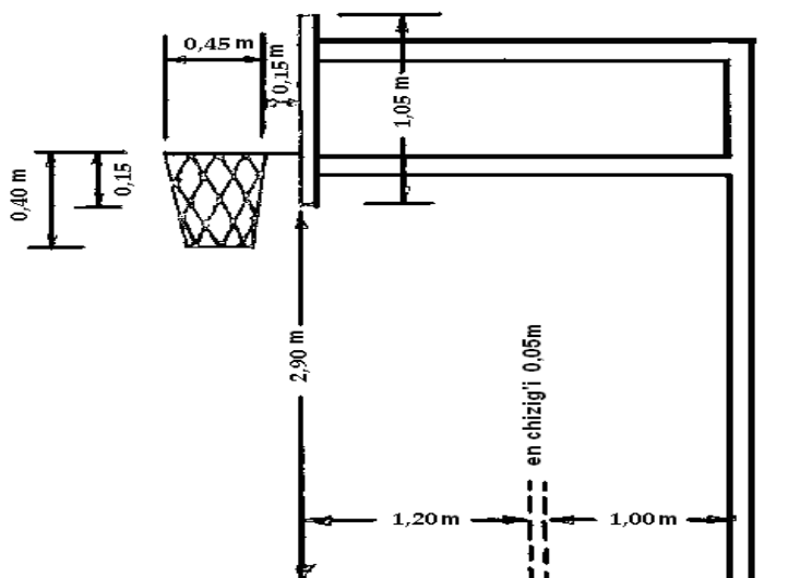
38-rasm. Halqa shit qurilmasi.
