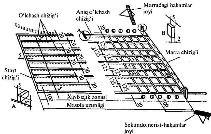
2-rasm. To'g'ri masofada alohida yo'lkalari bo'ylab hamma masofalar marralarining belgilanishi (o'lchamlar sm da ifodalangan).
